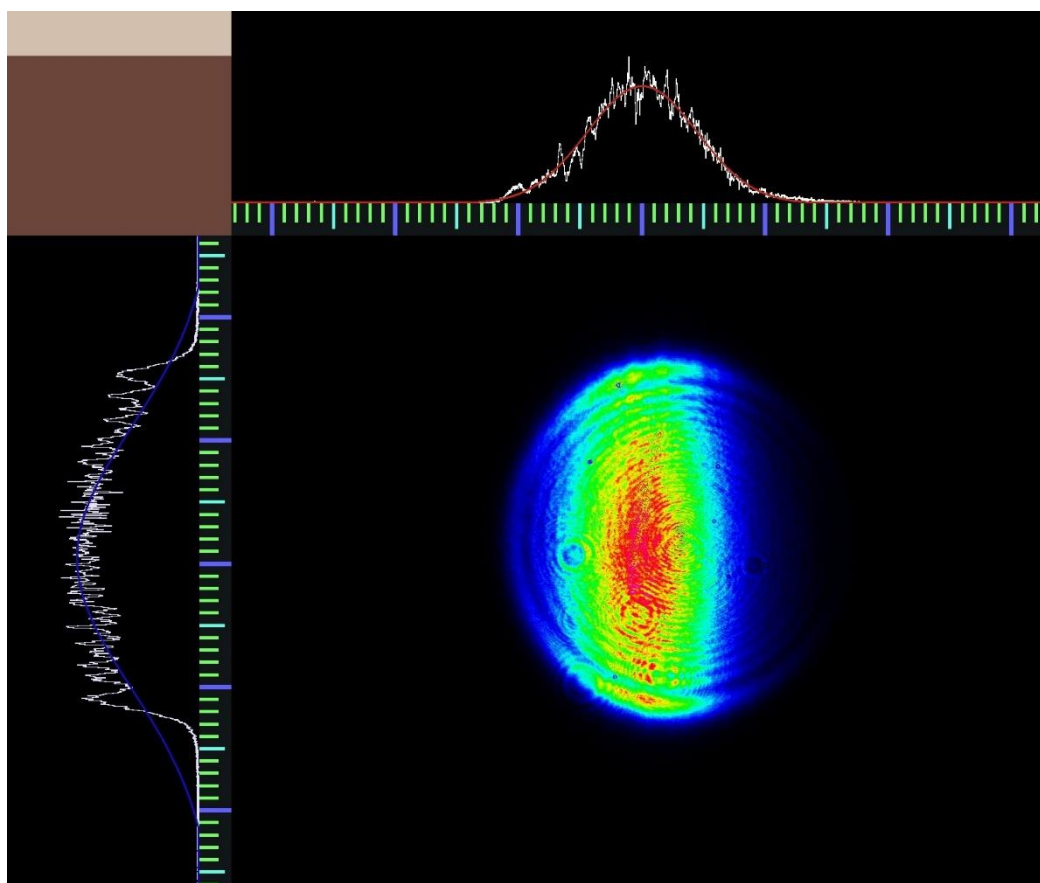
شکل ۱: پروفایل مازول لیزر ۵۲۰ نانومتر.
