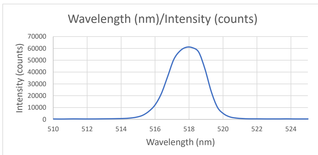
شکل ۲: طیف خروجی مازول لیزر ۵۲۰ نانومتر.
