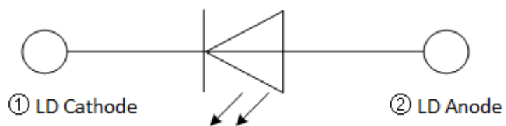
图 6-1 内部电路图
