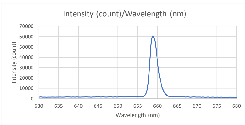
شکل ۲: طیف خروجی ماژول لیزر ۶۶۰ نانومتر.
