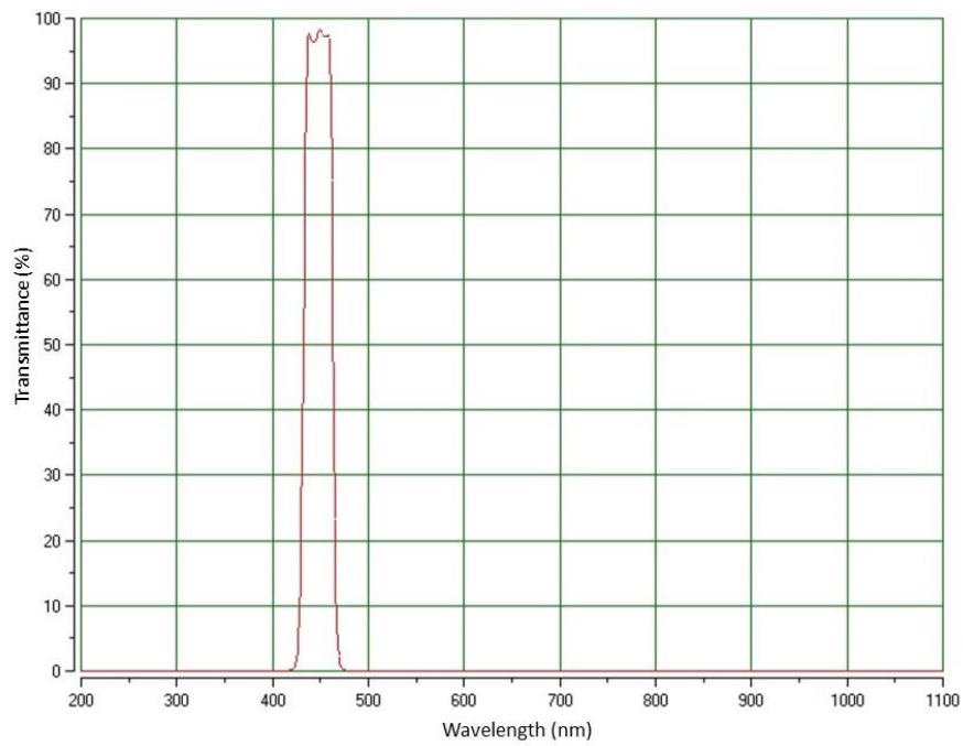
شکل ۱: نمودار درصد عبور برحسب طول موج برای فیلتر بندپس ۴۵۰ نانومتر.
