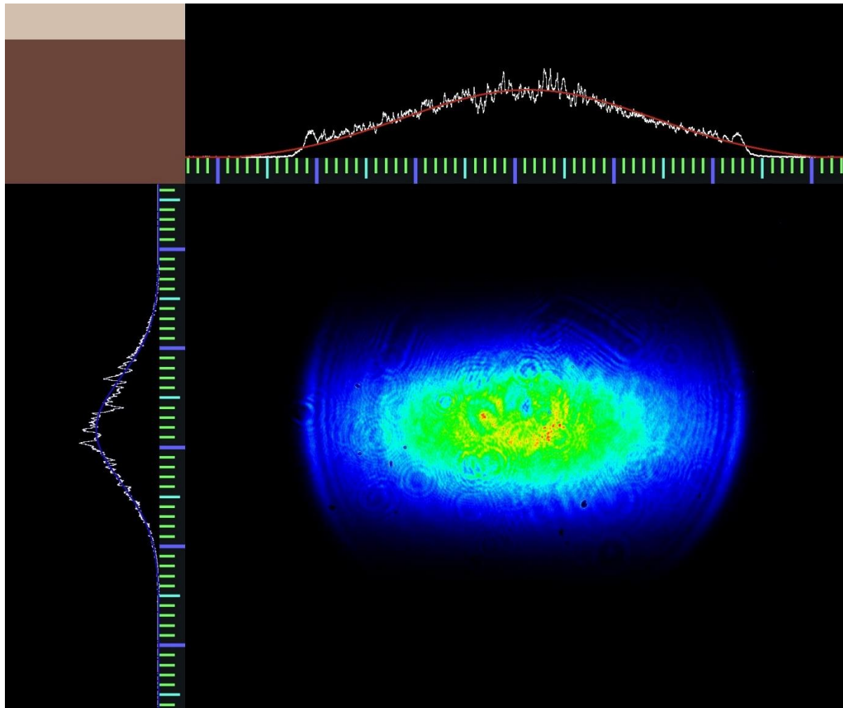
شکل ۳: پروفایل لیزر پوینتر ۴۰۵ نانومتر
